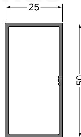
10563 0.585 Kg/m TUBO 50x25x1,5 mm.
