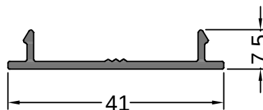
14422 0.212 Kg/m TAPA REFUERZO
