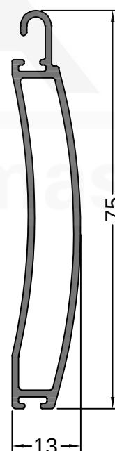
14336 0.558 Kg/m CORTINA ZOCALO PARA 12646
