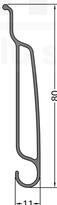
14440 0.554 Kg/m CORTINA PRIMERA TABLILLA
