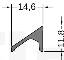
12448 0.135 Kg/m ABRIR GOTERON
