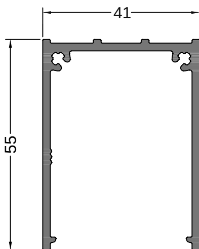
14421 0.886 Kg/m REFUERZO DE APLICAR
