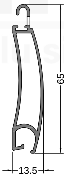
12352 0.499 Kg/m CORTINA TABLILLA CURVA MECANIZADA
