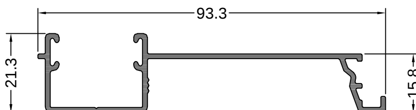
14129 0.587 Kg/m CORTINA GUIA COMUN 93.3 mm.
