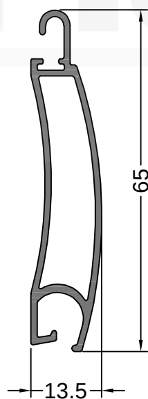
12646 0.499 Kg/m CORTINA TABLILLA CURVA
