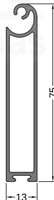
14442 0.655 Kg/m CORTINA ZOCALO PARA 14441
