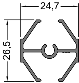
12232 0.309 Kg/m VIDRIO REPARTIDO NUCLEO
