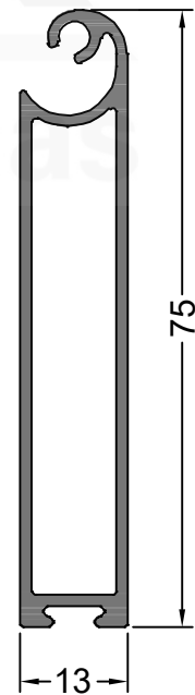
14442 0.655 Kg/m CORTINA ZOCALO PARA 14441
