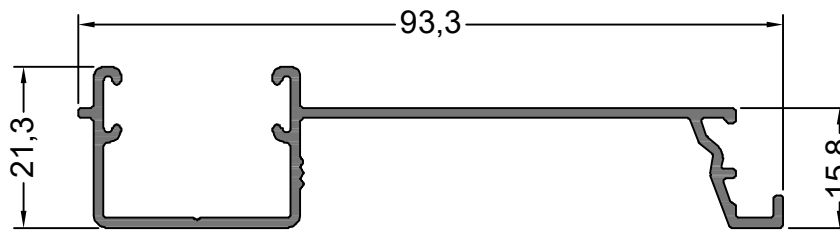
14129 0.587 Kg/m CORTINA GUIA COMUN 93.3 mm.
