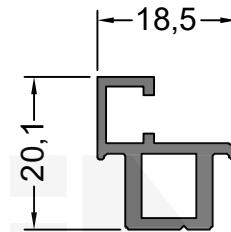
13332 0.273 Kg/m MOSQUITERO POSTIZO
