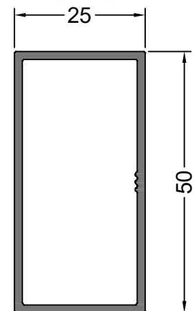
10563 0.585 Kg/m TUBO 50x25x1,5 mm.
