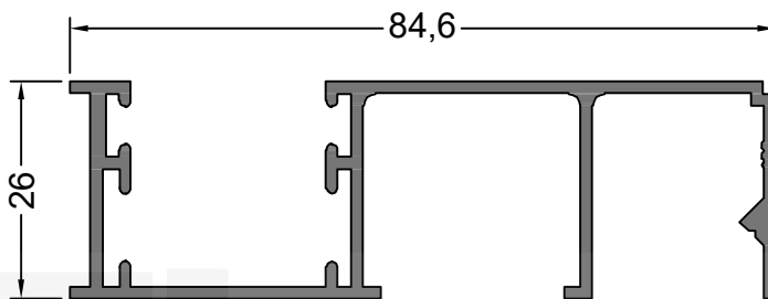
11648 0.847 Kg/m CORTINA GUIA COMUN 84.6 mm.
