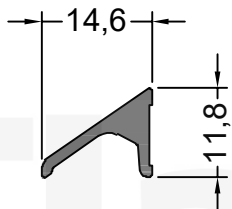
12448 0.135 Kg/m ABRIR GOTERON
