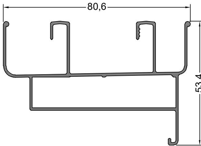
13345 0.903 Kg/m CORREDIZA MARCO UMBRAL CON TAPA JUNTA
