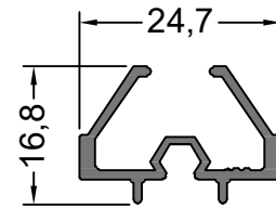
12249 0.232 Kg/m VIDRIO REPARTIDO PERIMETRAL
