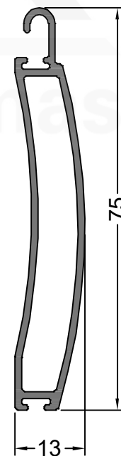
14336 0.558 Kg/m CORTINA ZOCALO PARA 12646
