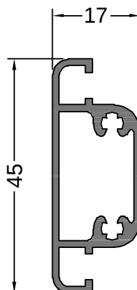
12693 0.492 Kg/m CORREDIZA MOSQUITERO TRAVESAÑO
