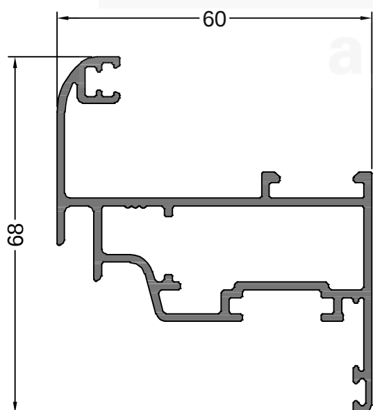
99852 1.104 Kg/m ABRIR HOJA
