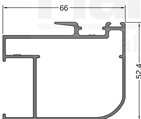
99882 1.103 Kg/m
