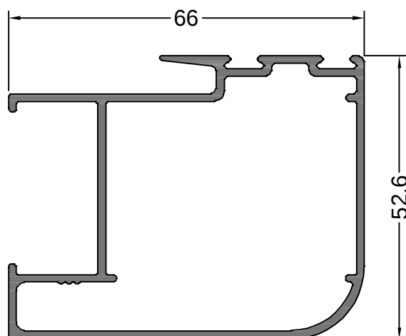
14589 1.080 Kg/m
