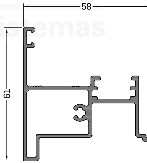
99844 1.036 Kg/m PUERTA ENCUESTRO 2 HOJAS
