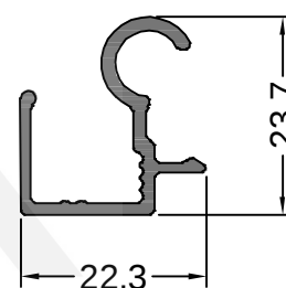
99254 0.272 Kg/m CORTINA BISAGRA
