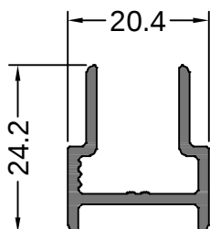
11747 0,289 Kg/m CORREDIZA ENCUENTRO 4 HOJAS
