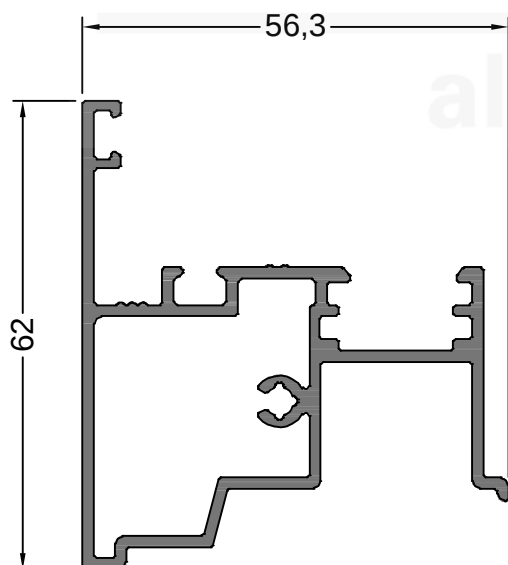
13164 1.059 Kg/m ABRIR ENCUESTRO 2 HOJAS
