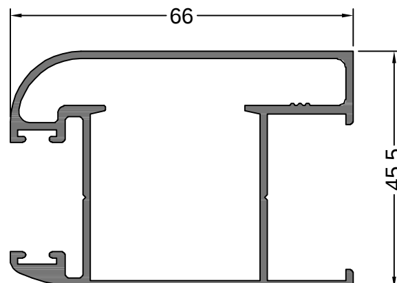
12138 1.101 Kg/m
